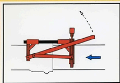
Startposisjon ved montering
